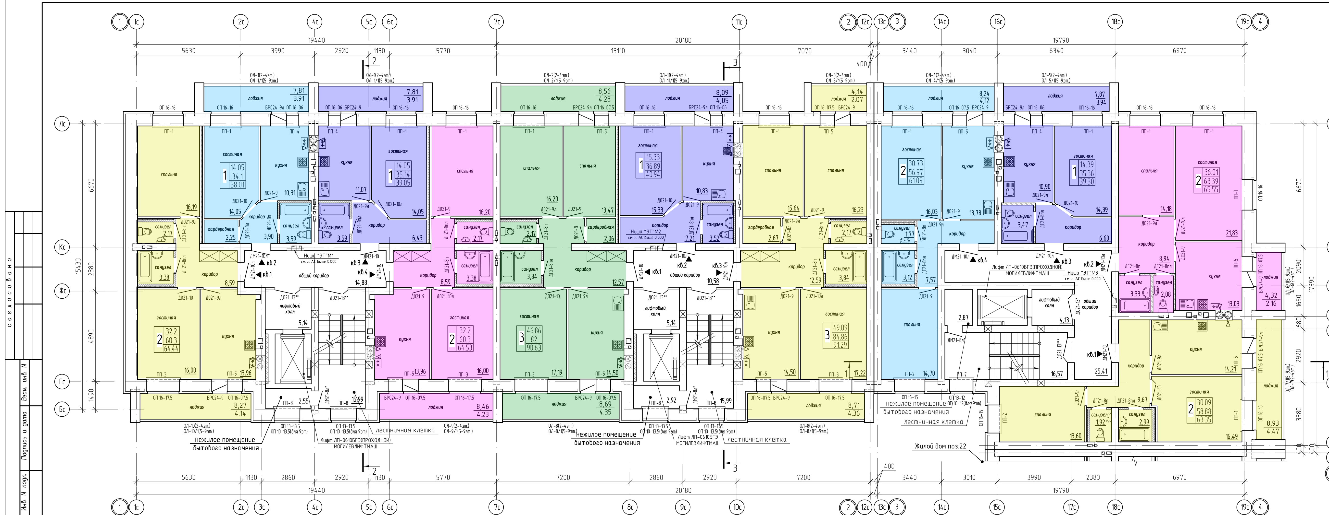
Показатели на типовой этаж в осях 1с-7с
